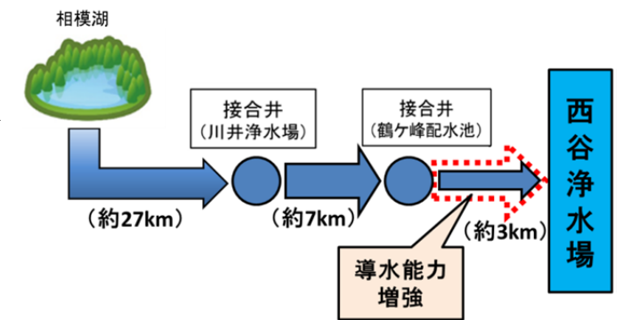
図 4 相模湖系導水路改良の概要
